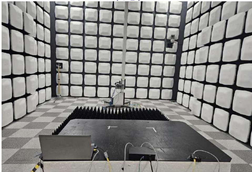
[ 후면 ]
