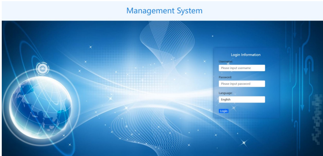
그림 1-4-1 로그인 창
