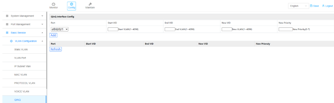
그림 4-1-7 QINQ 페이지
