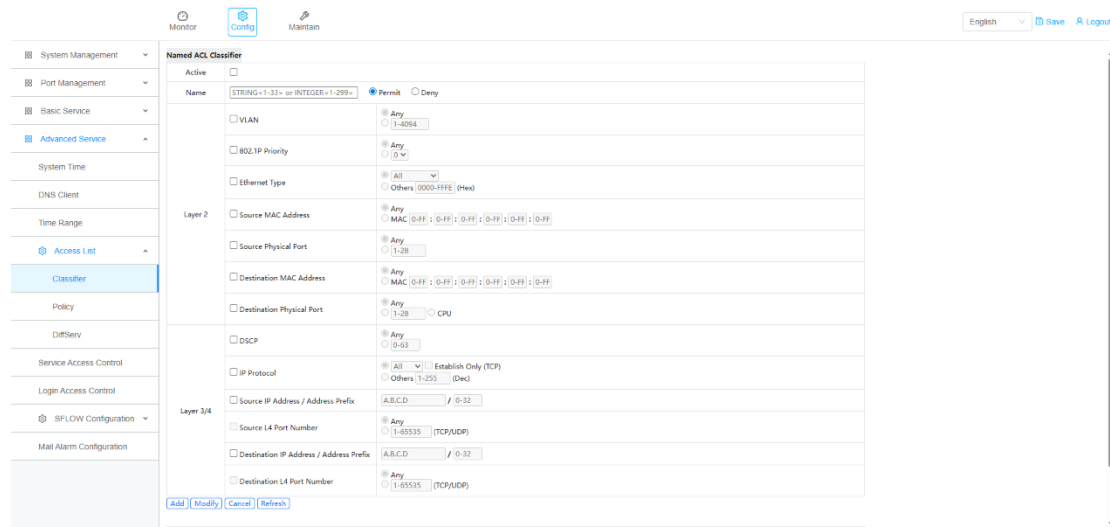
그림 5-3-1 분류기 페이지
