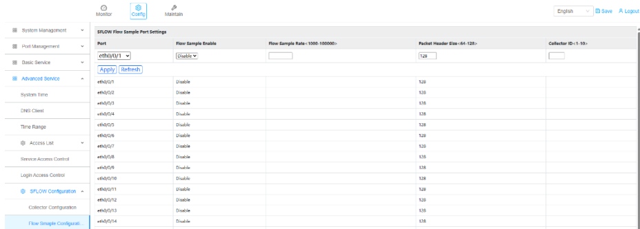
그림 5-5-2 플로우 스맵플 구성 페이지
