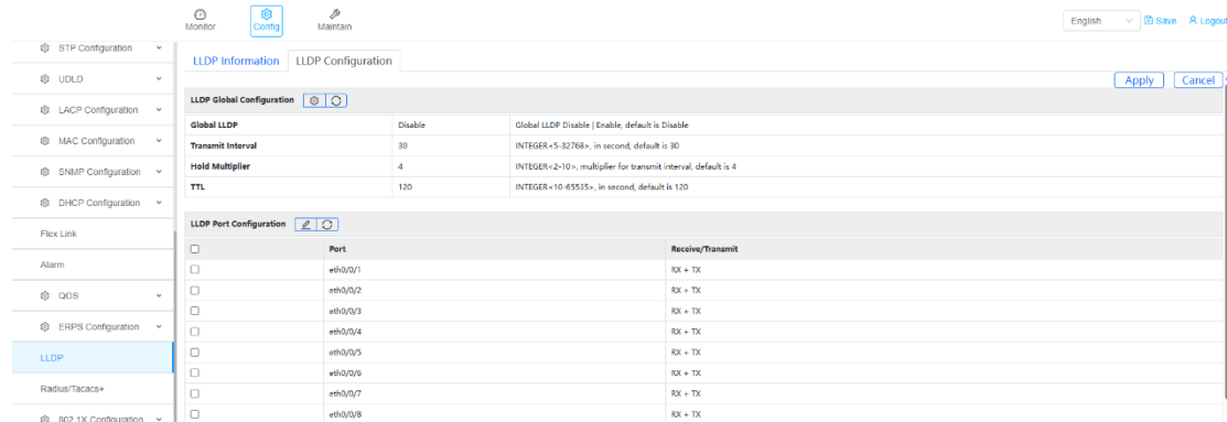
그림 4-17-2 LLDP 구성 페이지
