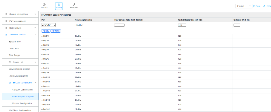
그림 5-6 우편 경보 구성 페이지
