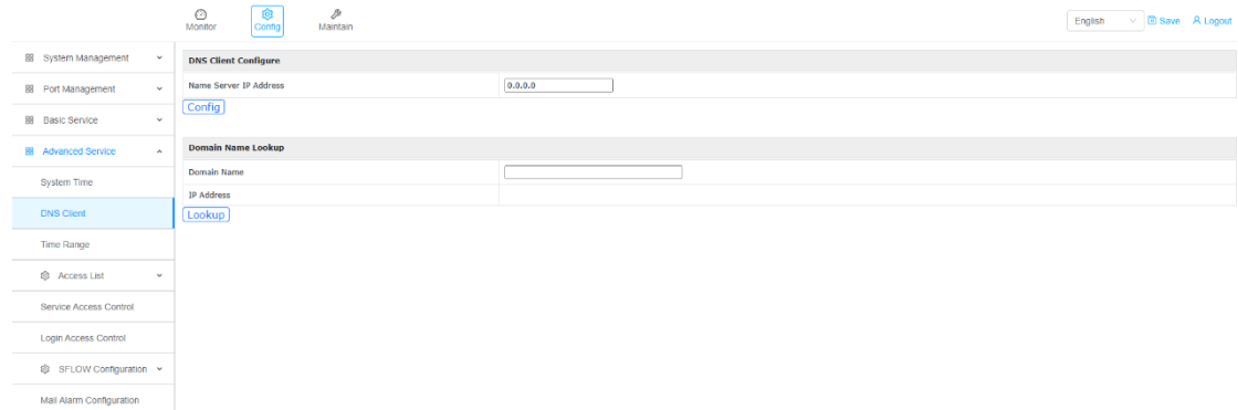
그림 5-1 DNS 클라이언트 페이지
