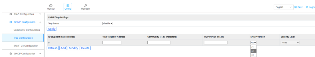
그림 4-11-2 트랩 구성 페이지
